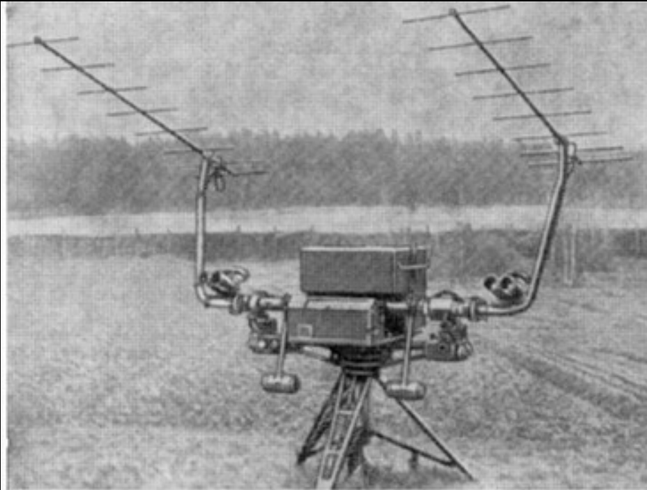
Зенитный радиодальномер «Хрусталь»
