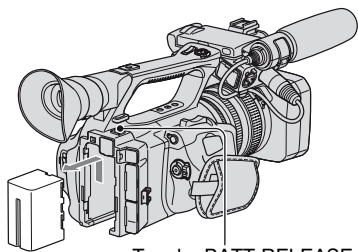
Touche BATT RELEASE (déblocage de la batterie)
